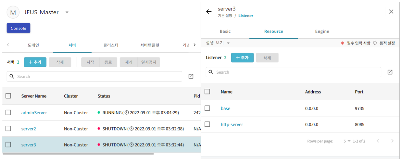
그림 12. HTTP 리스너 설정 - 리스너 추가
