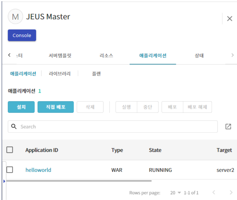
그림 25. Deployed Application 화면 - 웹 모듈 deploy 결과
