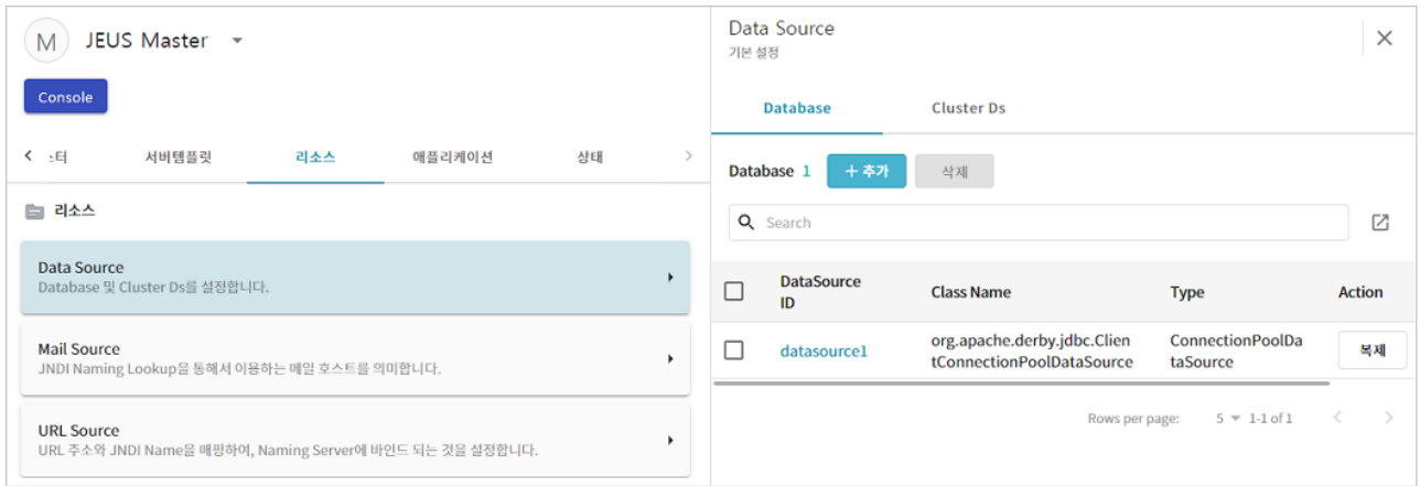
그림 18. 데이터소스 추가 - 목록 조회
