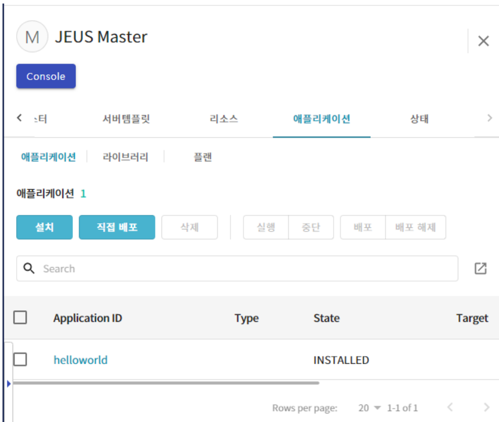
그림 23. 애플리케이션 화면 - 웹 모듈 설치 결과
