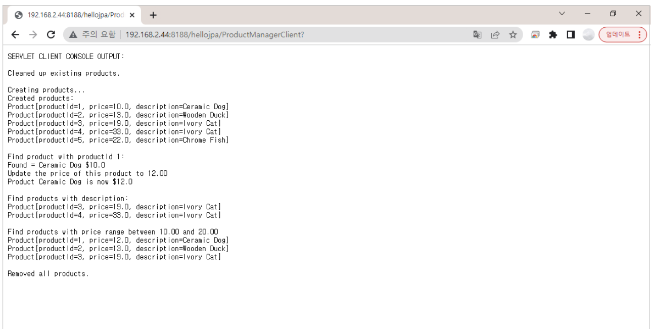
그림 41. HelloJPA 서블릿 클라이언트 수행 결과
