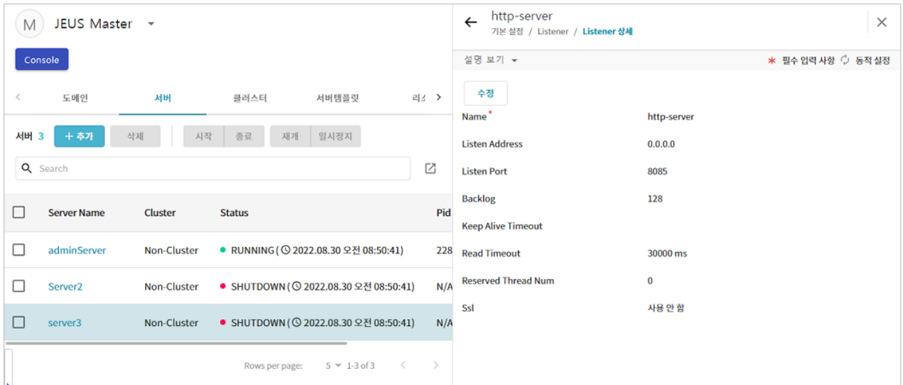
그림 11. MS 추가 - 리스너 설정 변경
